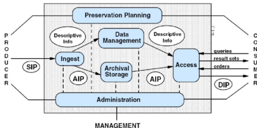
Figura 5 Modello OAIS di riferimento
