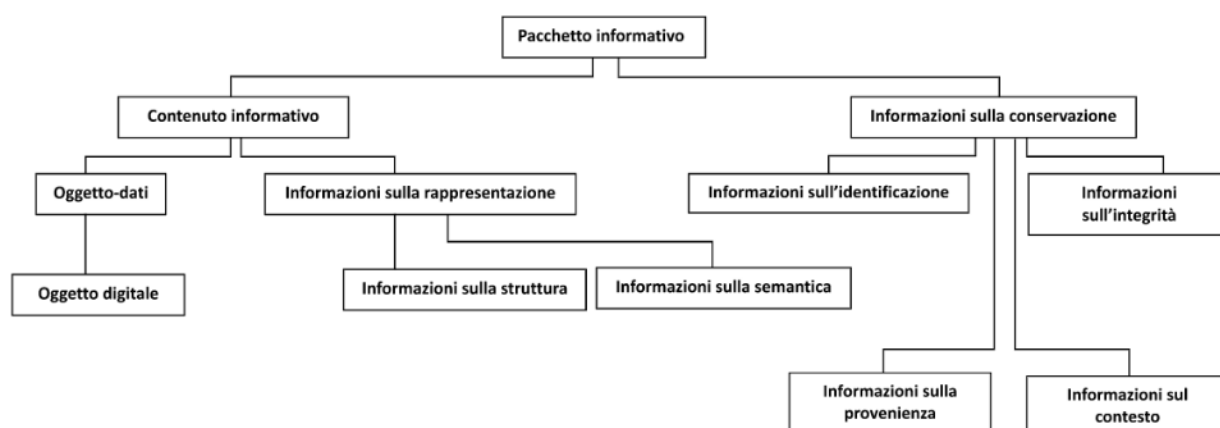
Figura. 3. Struttura di un pacchetto informativo
